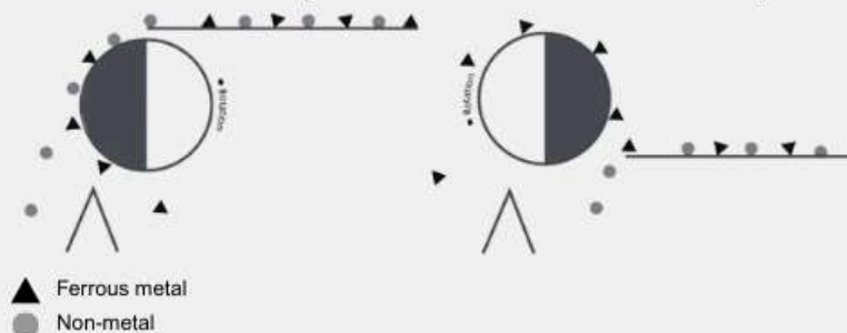
Obenbeschickter Trommelmagnet
